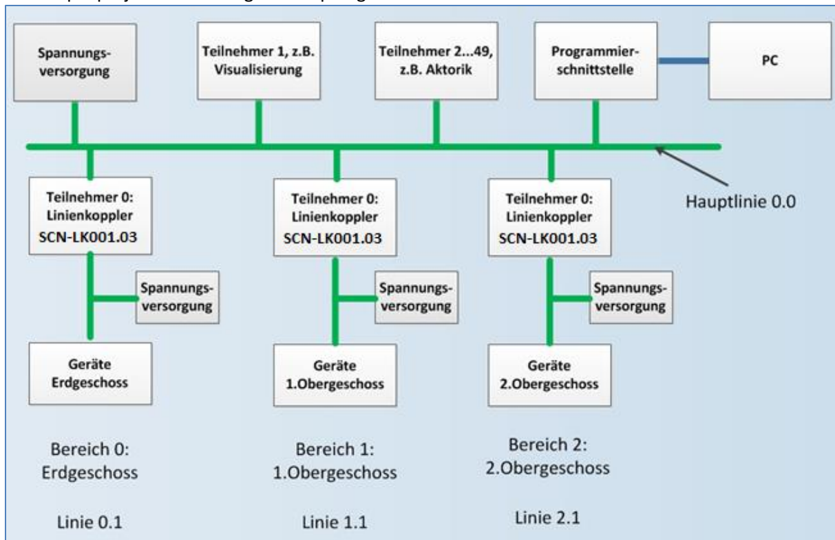
Abbildung 9: Topologie Beispielprojekt
