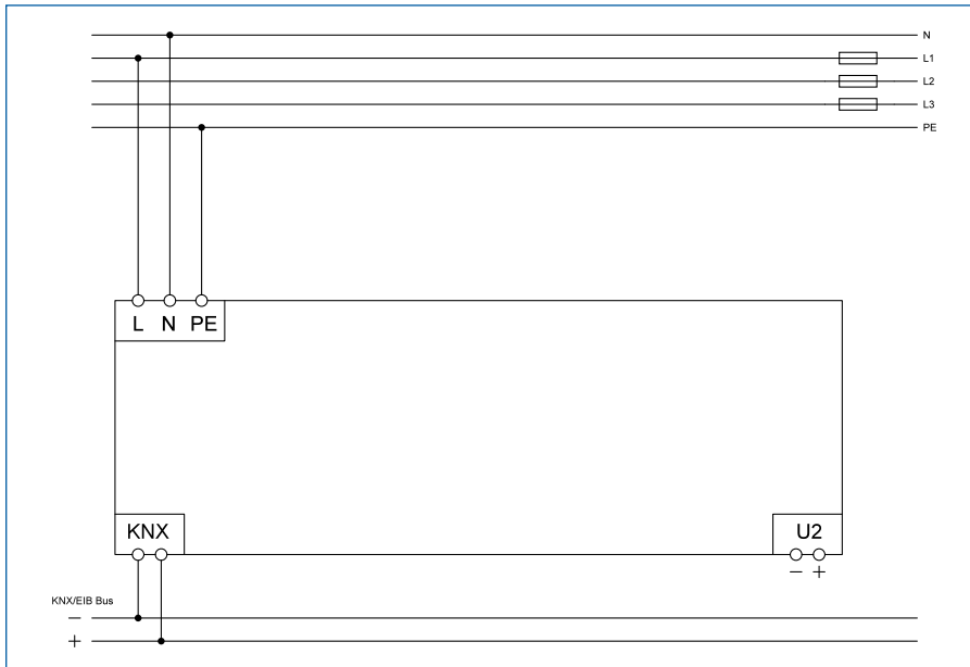
Abbildung 1: Anschlussschema
