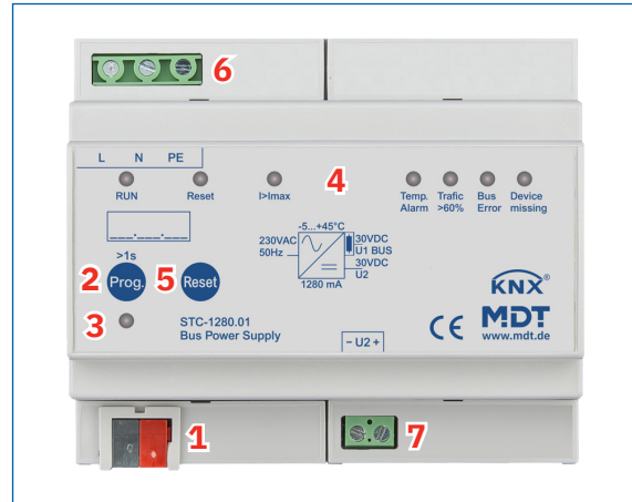
Abbildung 3: Aufbau und Bedienung: STC-0960.01 / STC-1280.01
