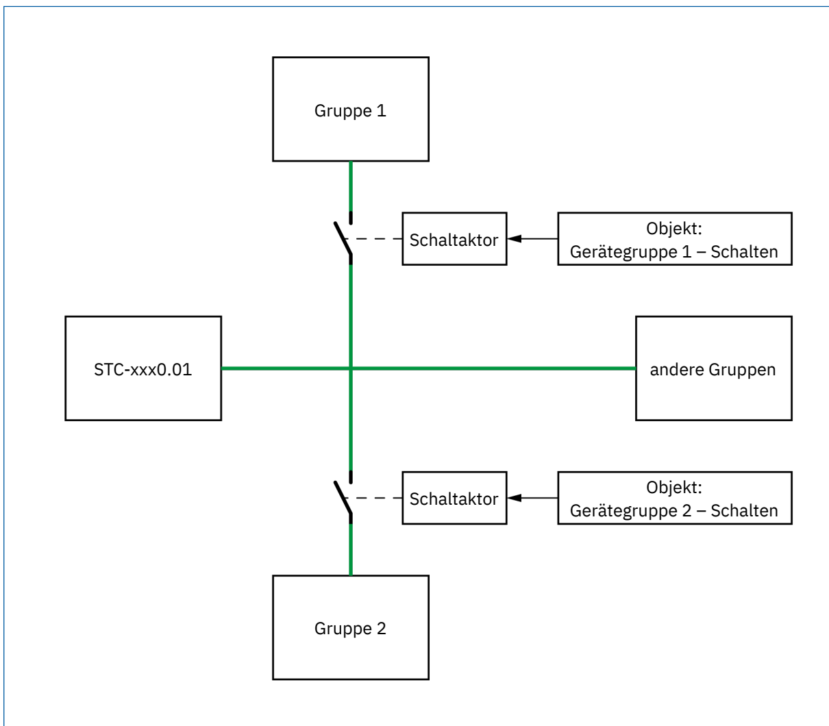
Abbildung 6: Diagramm – Topologie zur Trennung von KNX Teilnehmern
