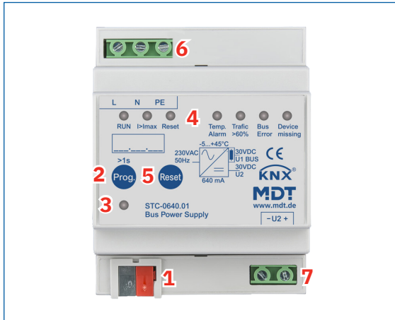
Abbildung 2: Aufbau und Bedienung: STC-0640.01
