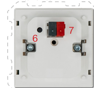
BE-TAL60xx.01 Back
