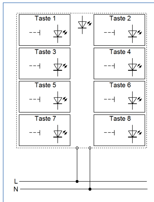
Abbildung 1: Anschlussbeispiel RF-TA55P8.01
