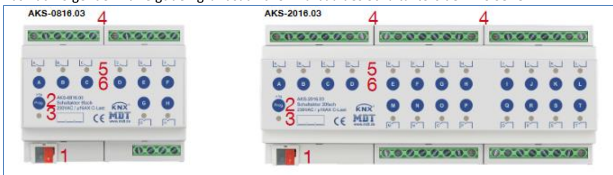
Abbildung 4: Aufbau & Bedienung – AKS Serie
