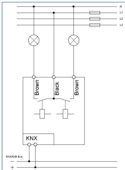
Abbildung 2: Anschlussbeispiel – AKS-02UP.03
