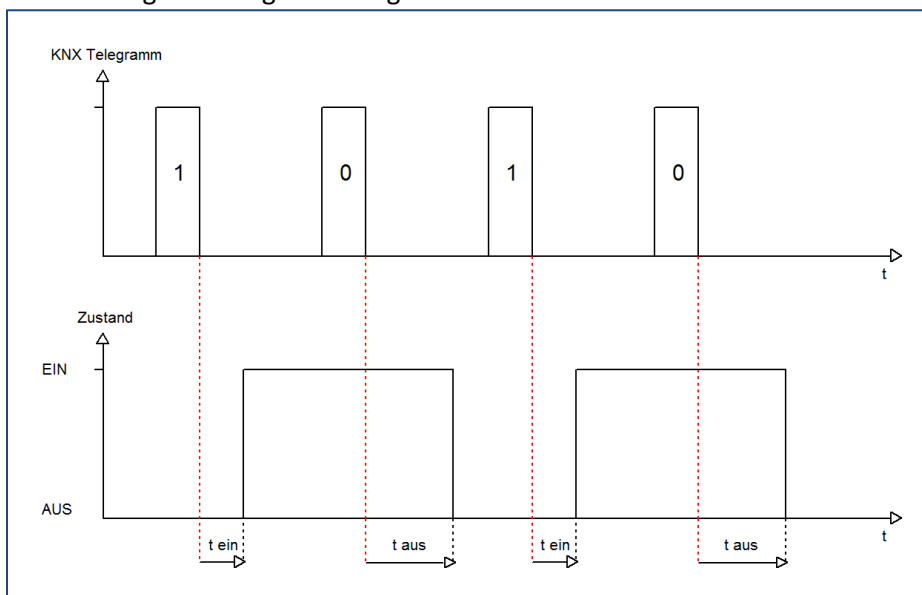
Abbildung 13: Ablaufdiagramm – Ein-/Ausschaltverzögerung
