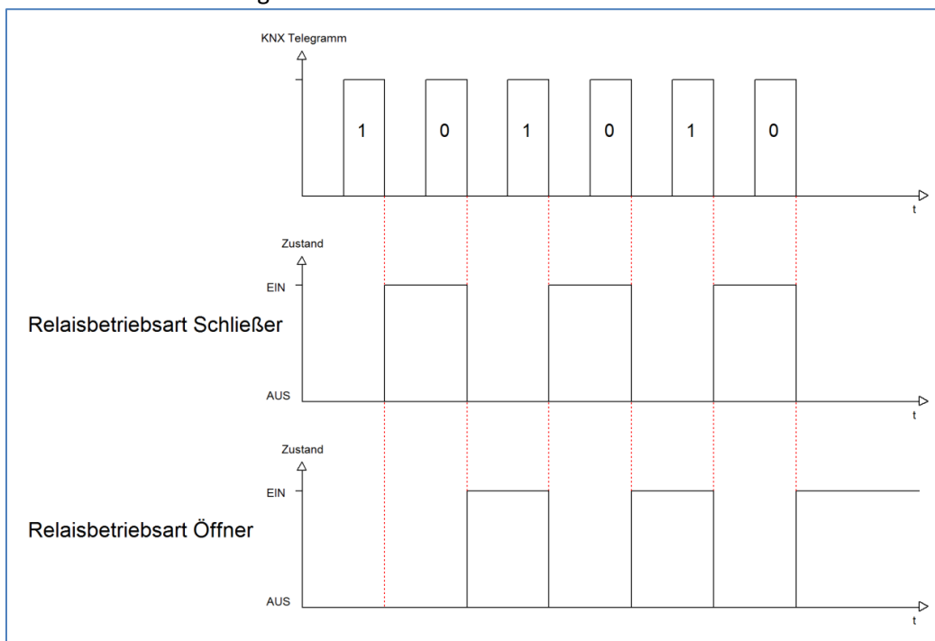
Abbildung 11: Ablaufdiagramm – Relaisbetriebsart
