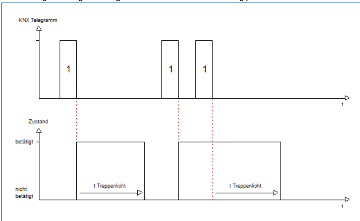
Abbildung 32: Ablaufdiagramm – Treppenlichtzeit verlängern
