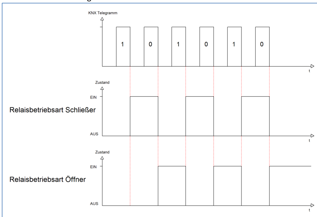
Abbildung 25: Ablaufdiagramm – Relaisbetriebsart
