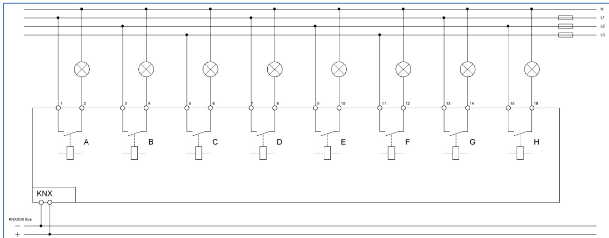
Abbildung 1: Anschlussbeispiel – AKx-0816.03
