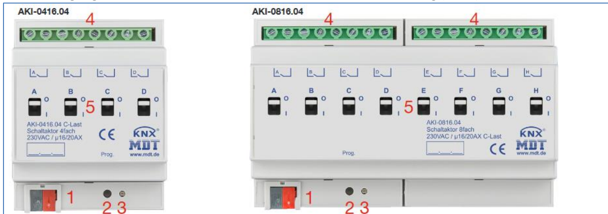
Abbildung 3: Aufbau & Bedienung – AKI Serie
