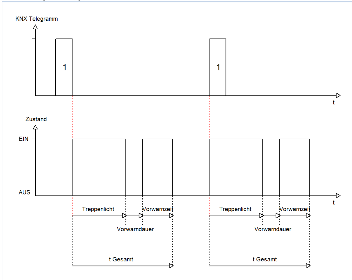
Abbildung 29: Ablaufdiagramm – Vorwarnung
